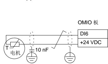
热敏电阻 (0)
